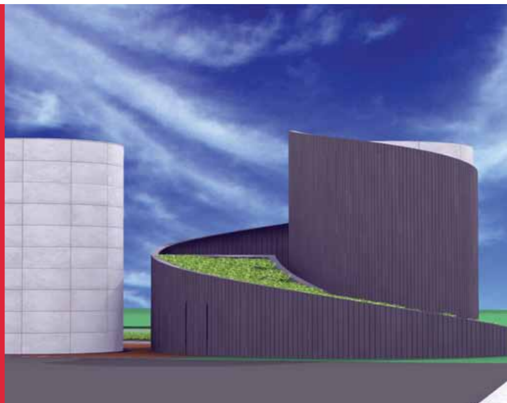
Een impressie van de centrale technische ruimte van Schuttersveld, waarin de warmte/koude opslag en het bluswater worden geregeld.
